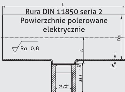
Rysunek wymiarowy EHG-DIN2-... / 1/2"
