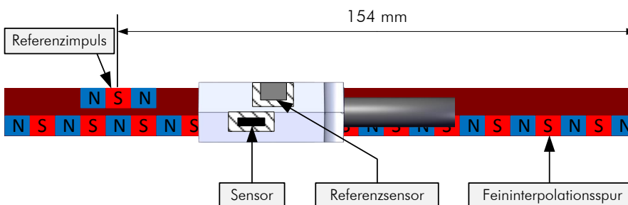
Abbildung 20: Übersicht Version 027
