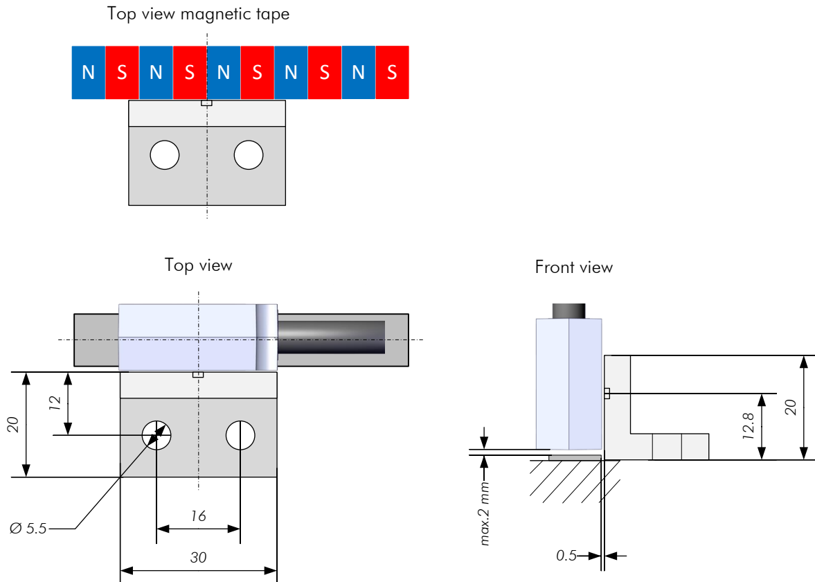
Abbildung 17: Montage des Magnetwinkels MW-007 für die Sonderausführung LMIX22-007
