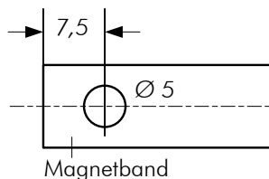
Abbildung 21: Magnetband mit Stanzlöchern
