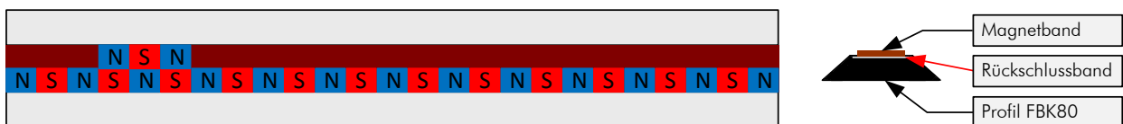
Abbildung 12: Magnetband-Varianten mit FBK80
