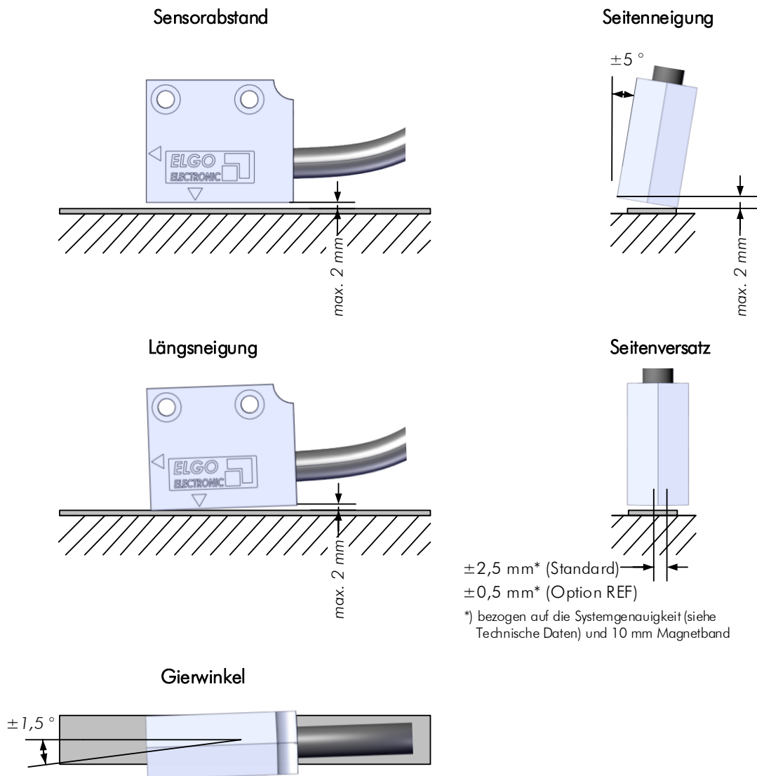
Abbildung 16: Toleranzen
