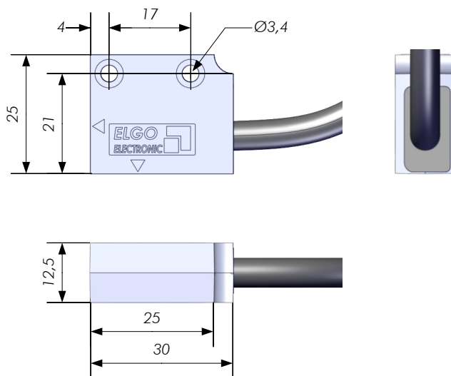
Abbildung 3: Abmessungen LMIX22
