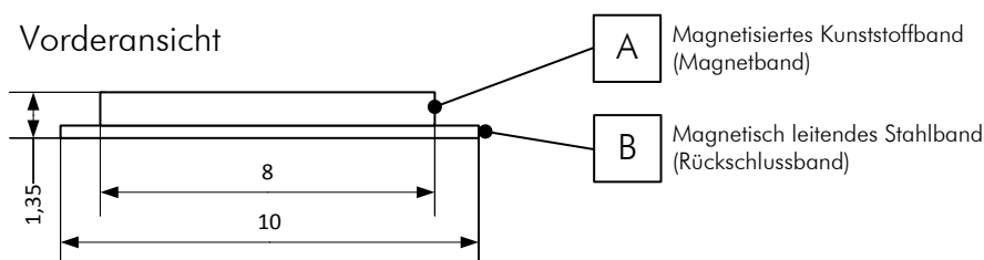
Abbildung 9: Magnetband MB20-20-10-1(2)-R-D-BK80
