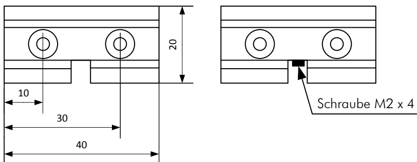
Abbildung 5: Abmessungen AFBK 80
