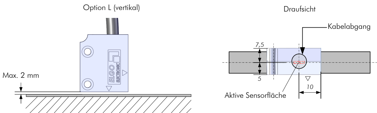
Abbildung 15: Montage der vertikalen Ausführung (Option L)
