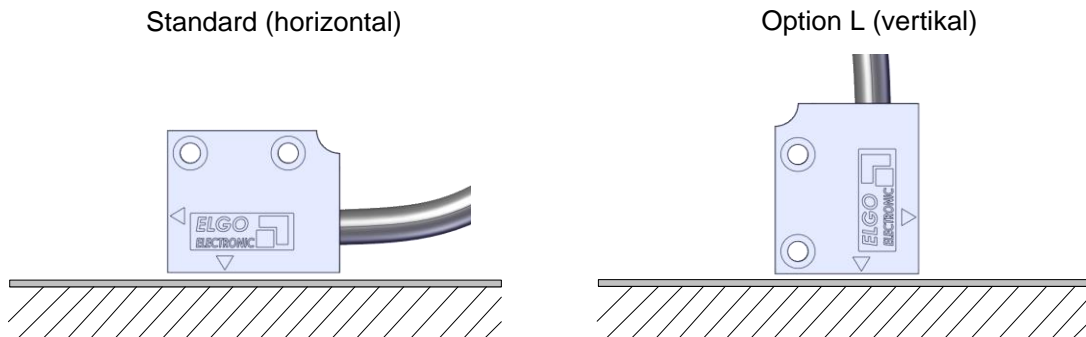
Abbildung 13: Montagemöglichkeiten des Sensors
