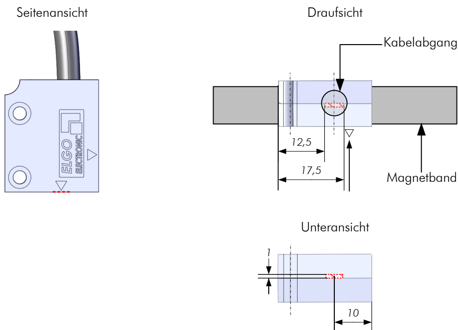
Abbildung 7: Vertikale Sensorposition (Option L)
