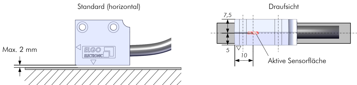
Abbildung 14: Montage der Standardausführung
