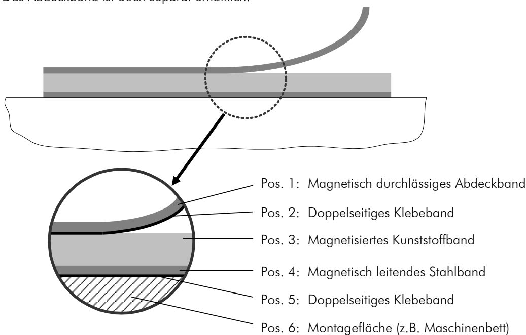
Abbildung 8: Magnetbandaufbau
