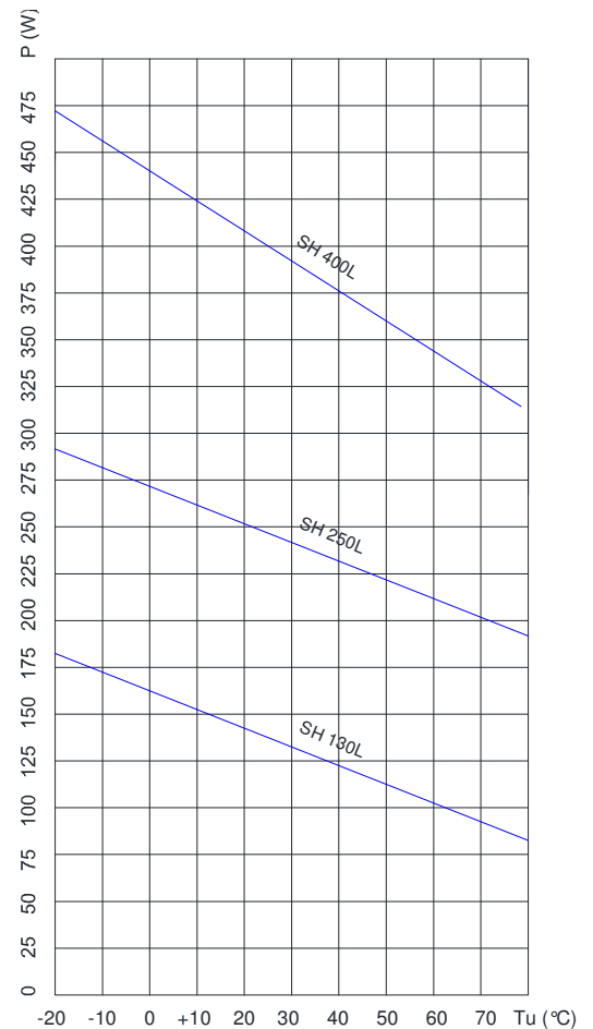
Leistung in Abhängigkeit von der Umgebungstemperatur Thermal output depending upon ambient temperature
