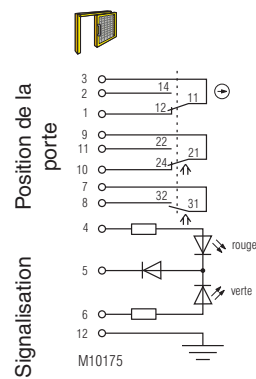
Fig. 2 : Verrouillage à l'état désactivé: actionneur retirés, porte ouverte
