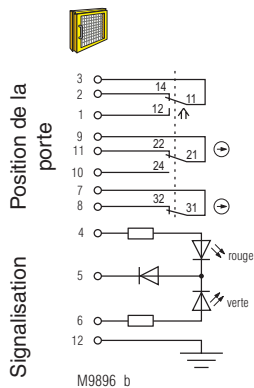
Fig. 1 : Verrouillage à l'état activé: actionneur insérés, porte fermée
