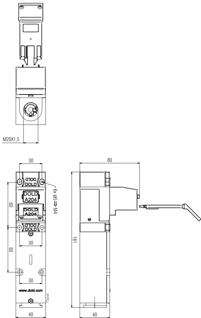
SX01M Tolérances générales ± 2%
