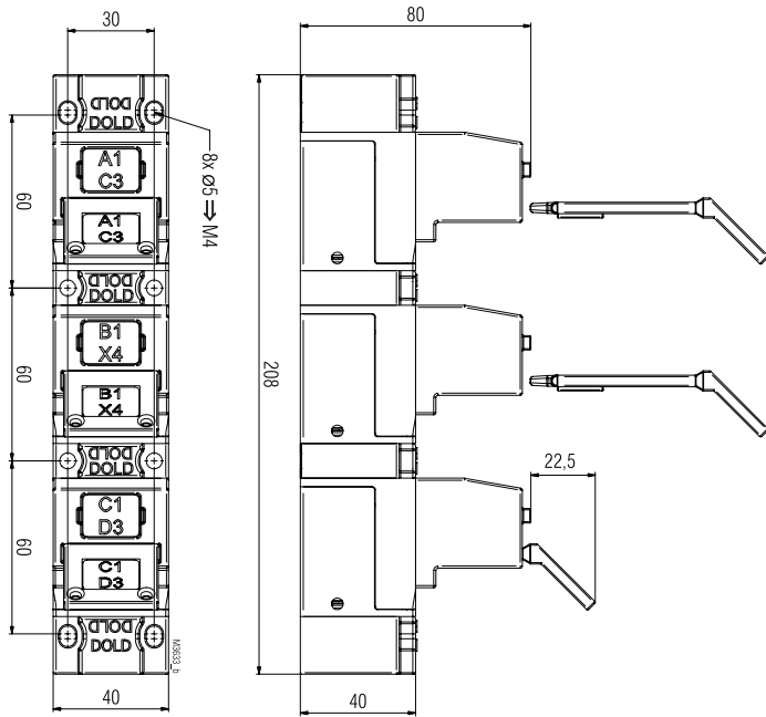
Abbildung: M12M Freimaßtoleranzen ± 2%
