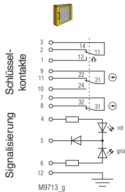
Bild 1: Verriegelung im aktivierten Zustand: 1. Schlüssel entnommen, Betätiger gesteckt, 2. Schlüssel gesteckt, Tür geschlossen
