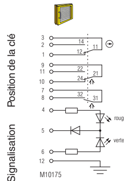
Fig. 2 : Verrouillage à l'état activé: 1 re Clé retirée, actionneur insérée, 2 e Clé insérée, porte fermée
